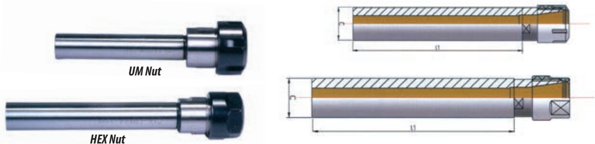
HEX Nut
