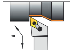
MDJNR
